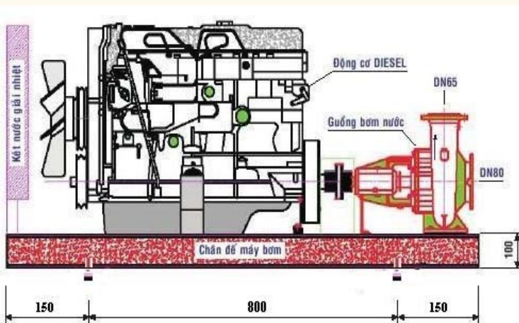
MẶT CẮT DỌC
